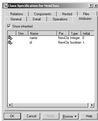
Рисунок 5.10. Добавление атрибута в окне спецификации класса.
