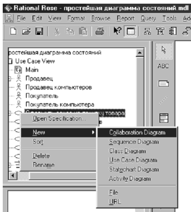
Рисунок 4.2 Создание новой диаграммы кооперации.
