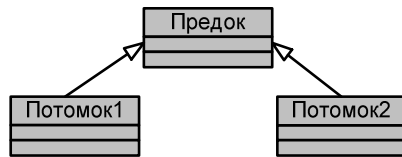
Рисунок 5.21. Отношение обобщения.
