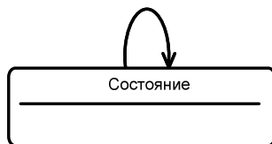
Рисунок 3.5. Рефлексивный переход.
