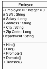
Рисунок 5.12. Пример класса, видимость атрибутов которого выполнена в нотации UML.
