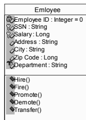
Рисунок 5.13. Пример класса, видимость атрибутов которого выполнена в нотации Rational Rose.
