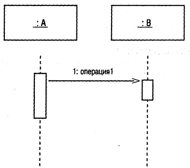
Рисунок 5.16. Фрагмент диаграммы взаимодействия.
