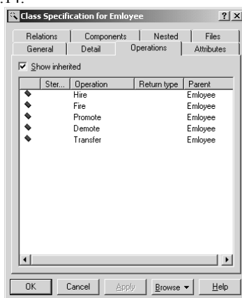
Рисунок 5.14. Добавление новой операции в окно спецификации класса.
