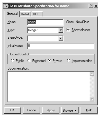
Рисунок 5.11. Окно спецификации атрибута.
