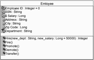
Рисунок 5.15. Добавление аргументов к операции.
