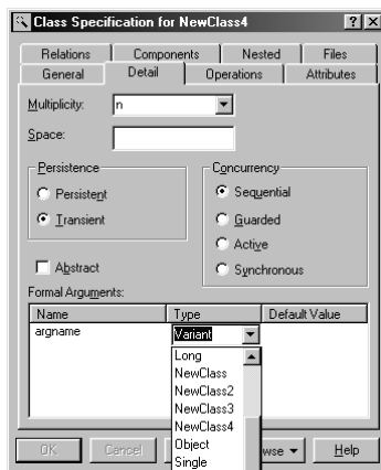
Рисунок 5.4. Задание аргументов параметризованного класса.
