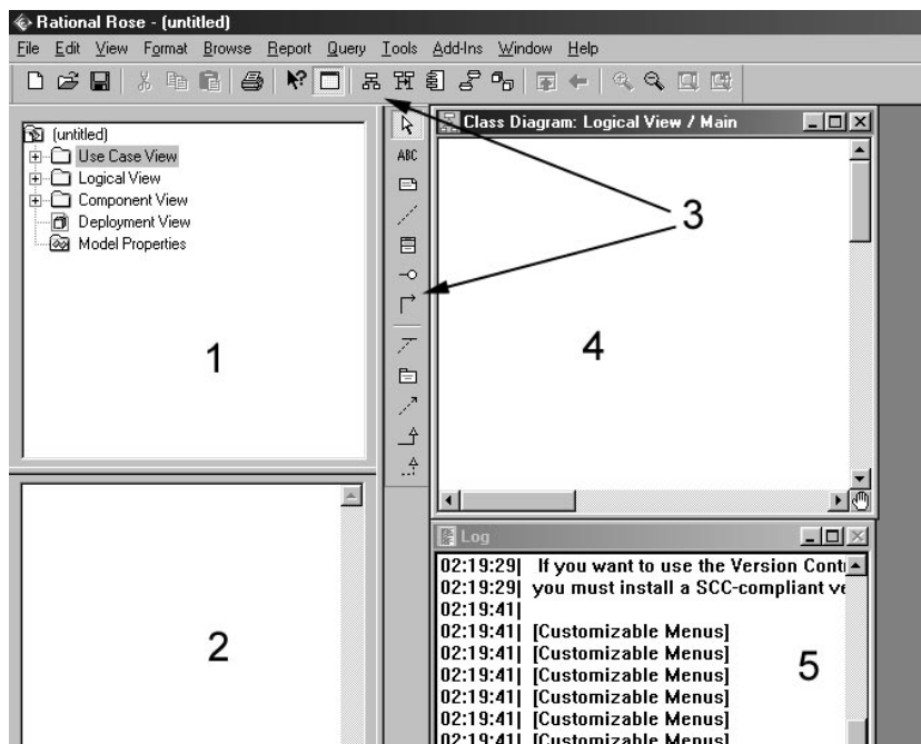
Рисунок 1.3. Основные элементы интерфейса Rational Rose 2002
