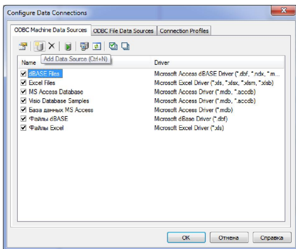
Рис. 21. Окно конфигурации ODBC
