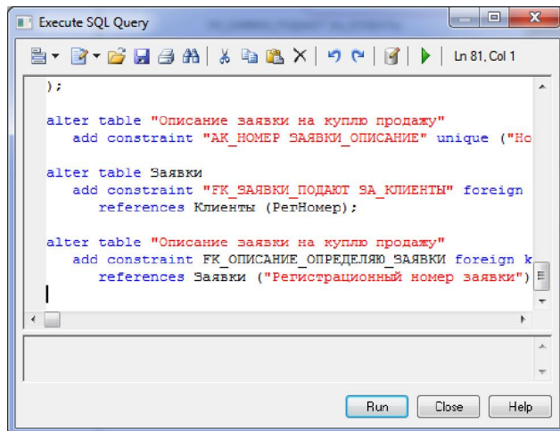
Рис. 27. Окно SQL-скрипта на создание схемы БД
