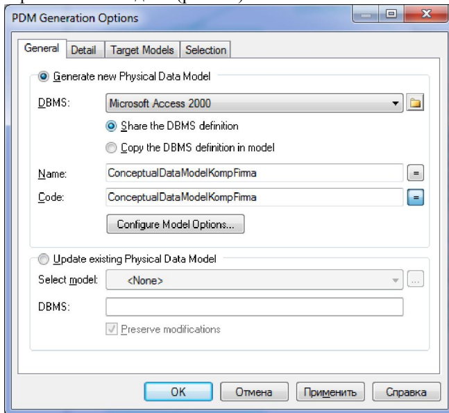
Рис. 16. Окно генерации физической модели
